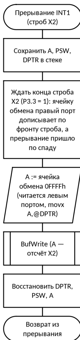
Рис. 6. Схема алгоритма: Обработчик прерывания INT1: приём отсчёта X2 от внешнего устройства
